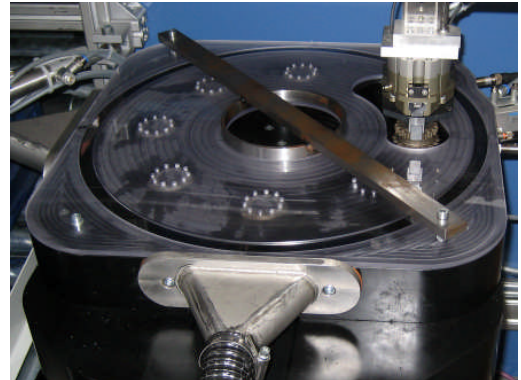
Bild 3: Reinigung rotationssymmetrischer Werkstücke in einem liegenden Revolver.
