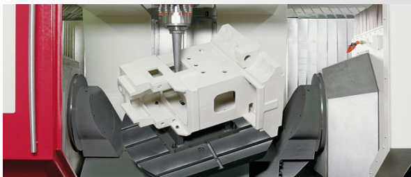
Fräsen eines Gussgehäuses
